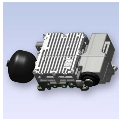
Versnellingsbakactuatoren
