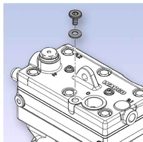
Închiderea portului 4 a compresorului
