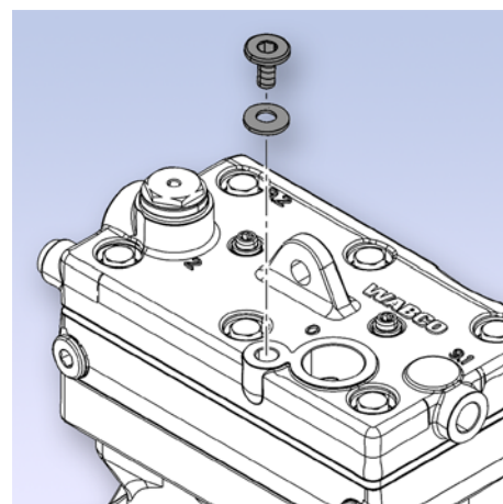
Chiudere il collegamento 4 dal compressore
