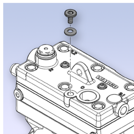
A 4-es csatlakozó pont lezárása a WABCO kompresszoron
