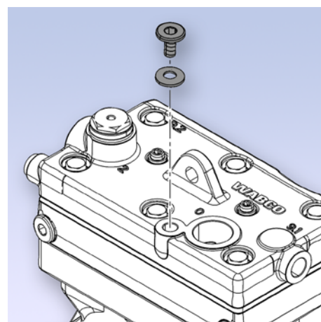
Затваряне на порт 4 на компресора
