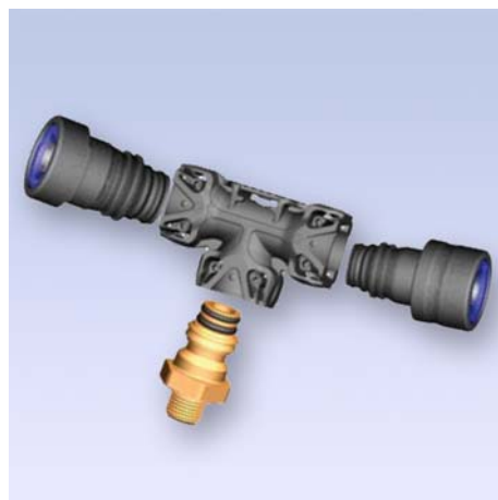
Пример сборки системы элементов сборной конструкции из композитов
