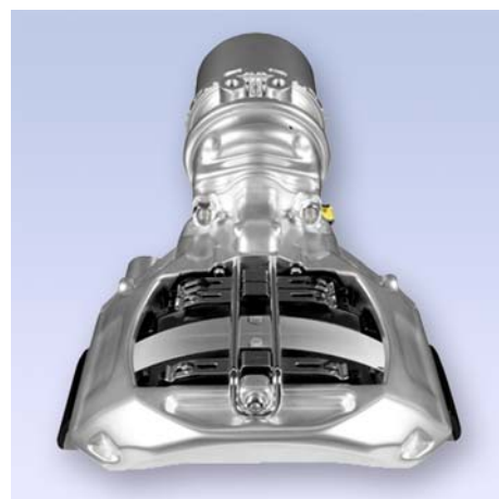
Сверхмощный пневматический дисковый тормоз MAXX 22
