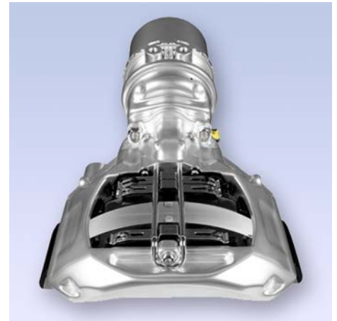
Frenos de disco neumáticos MAXX 22
