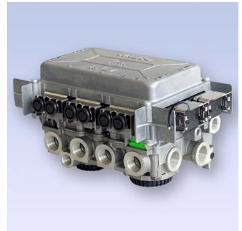
Modulador TEBS D REMAN
