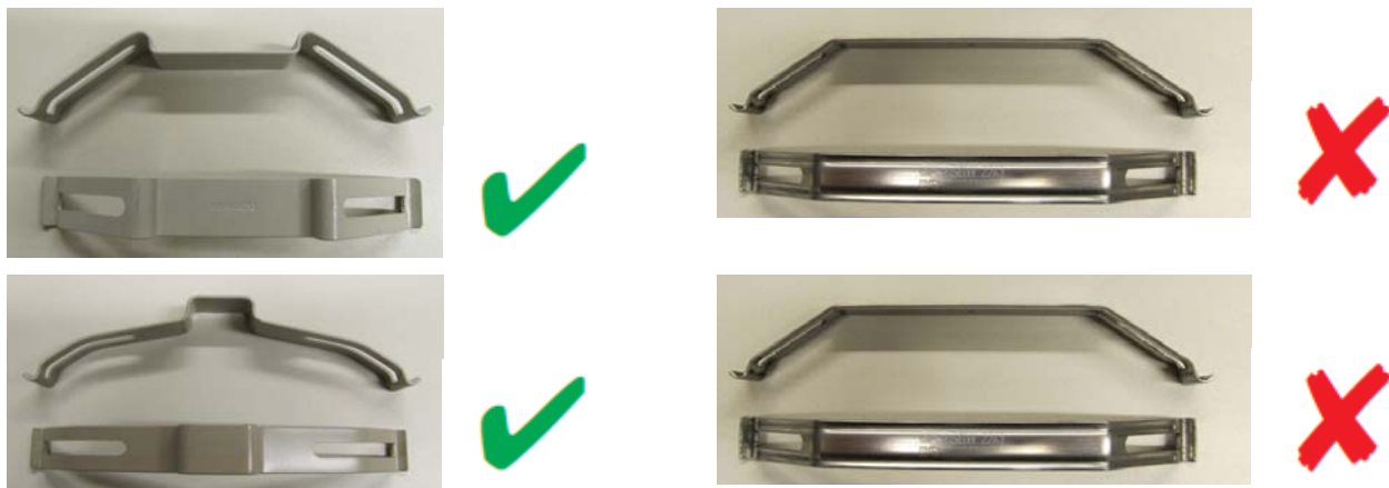
WABCO Original-Niederhaltefedern
