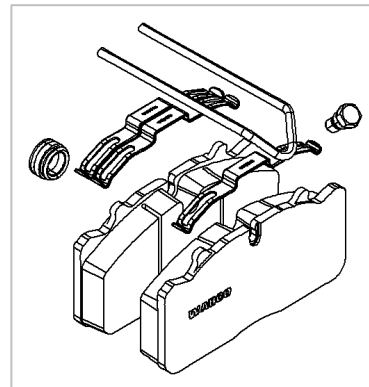
Fig. 1: kit di riparazione WABCO
