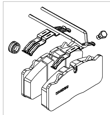
Fig. 1: Conjunto de reparación WABCO
