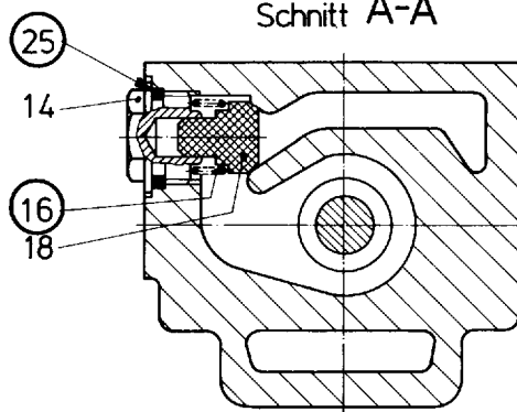
Schnitt A-A
