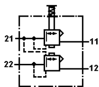
Fig. 1 + 2 Distributore di comando veicolo a motore 461 315 ... 0, simbolo di funzione
