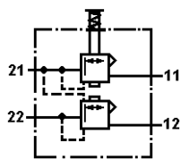
Abb. 1 + 2 Motorwagen-Bremsventil 461 315 ... 0, Funktionssymbol
