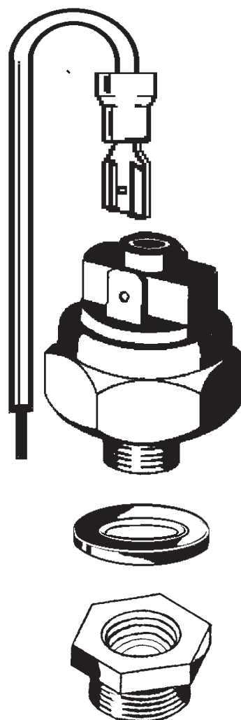
Contact de la masse par le fil à raccorder au chassis
