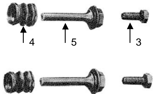
Reparatursatz Führungsbolzen
