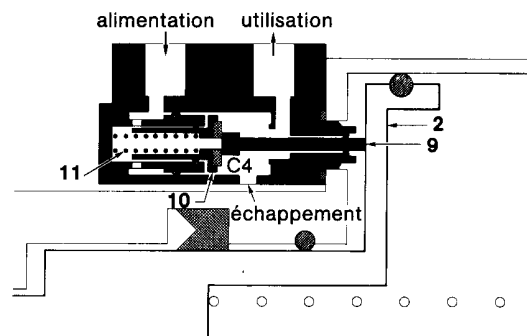
figure 4 - position embrayée
